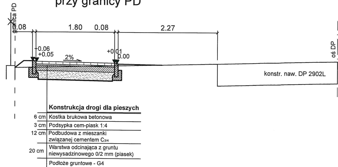
Przekrój przez peron i drogę dla pieszych
