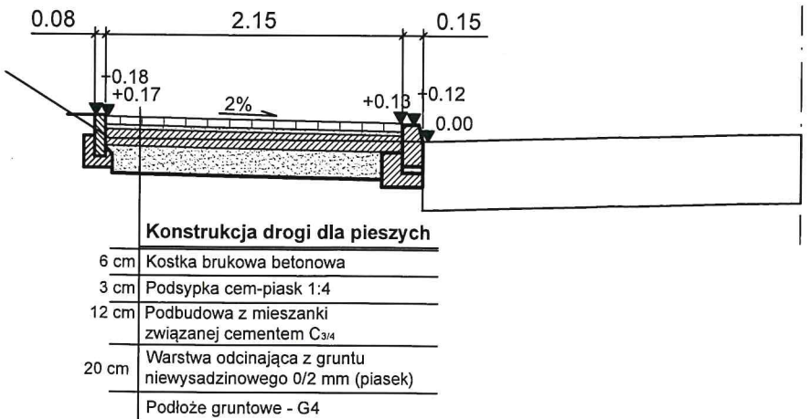
Przekrój typowy przez drogę dla pieszych przy krawędzi jezdni
